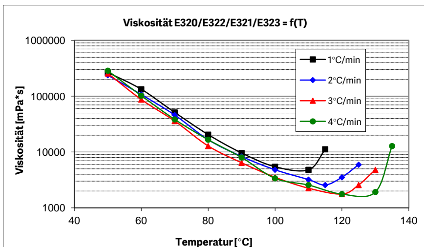
Abb. 2: Viskosität von E320/E321/E322/E323 in Abhängigkeit der Aufheizrate
