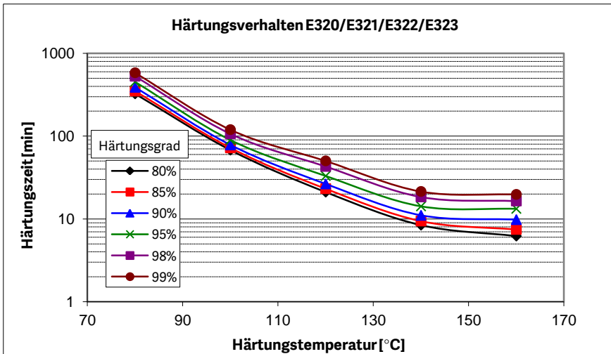
Abb. 1: Zeit/Umsatzkurven von E320/E321/E322/E323
